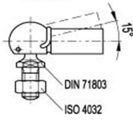
DIN 71802-CS
