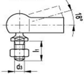
DIN 71802-C
