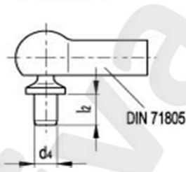
DIN 71802-B
