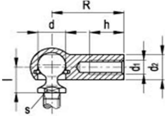
DIN 71802-C
